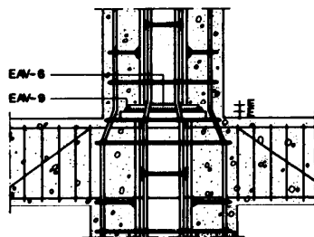
Alzado
