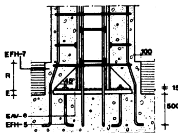
Alzado
