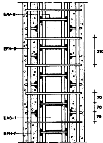
Alzado
