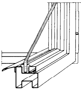
Sección horizontal
