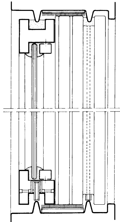
Sección vertical
