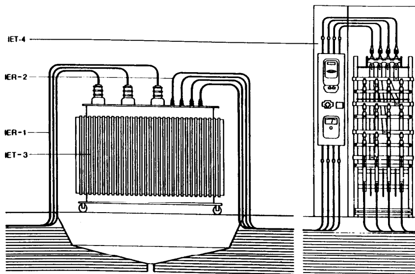
Sección
