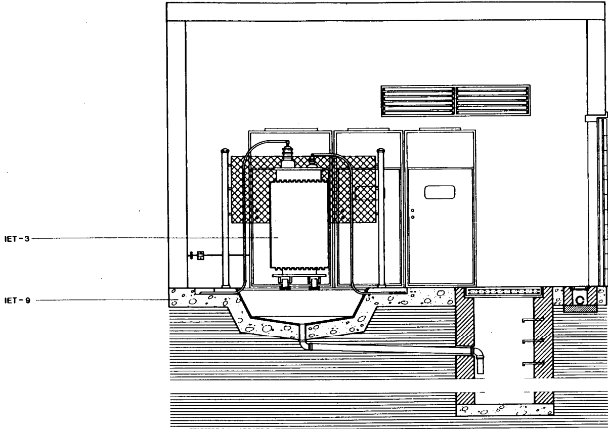
Sección
