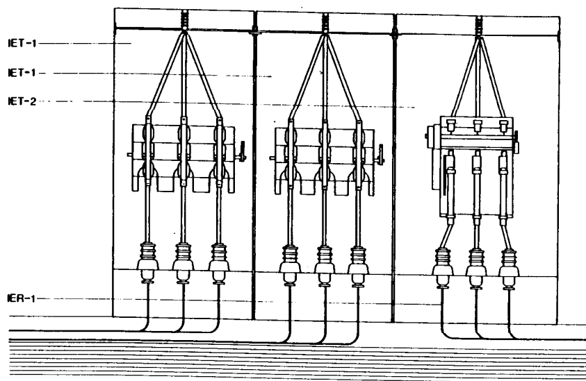
Sección
