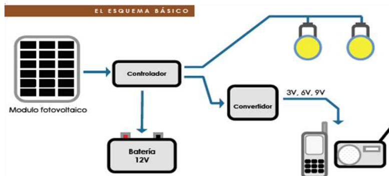
Esquema de instalación del Sistema Fotovoltaico
