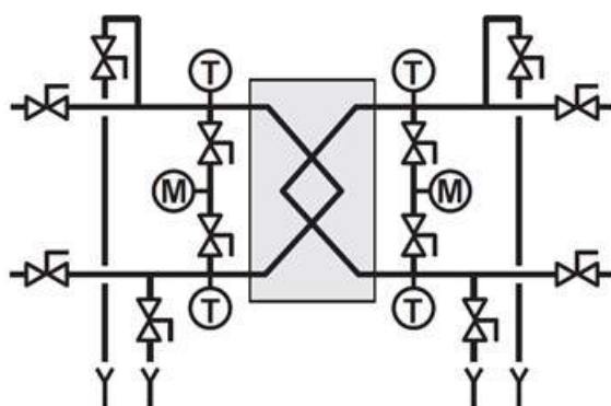
Figura 72: Esquema (izq.) y ejemplo (der.) del conexionado de un intercambiador solar independiente
