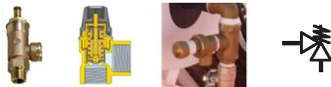
Figura 76: Ejemplo de válvula de seguridad, esquema, instalada y símbolo habitualmente utilizado
