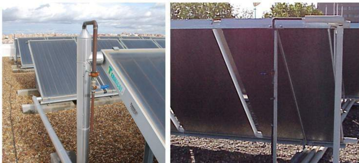
Figura 102: Ejemplos de purgadores de aire manuales y con escapes conducidos
