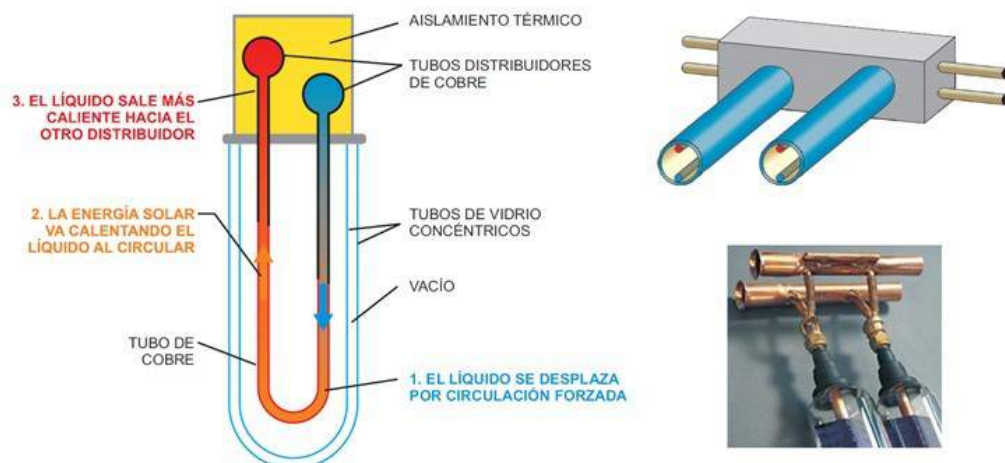
Figura 21: Captador de tubos de vacío con “tubo en U” y con “tubos concéntricos”
