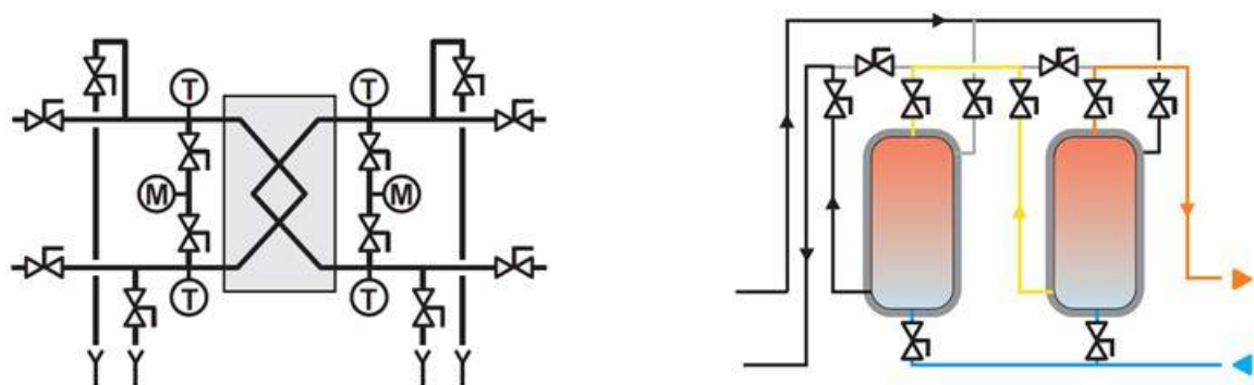
Figura 90: Ejemplos de esquemas de subsistemas con intercambiador independiente y un conjunto de dos acumuladores conectados en serie
