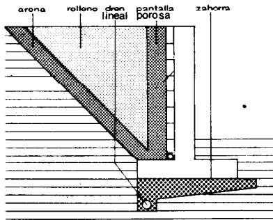
Sección vertical
