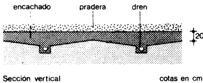
Sección vertical
