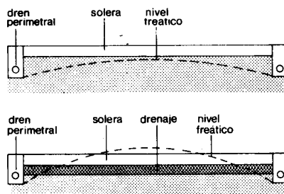
Secciones verticales
