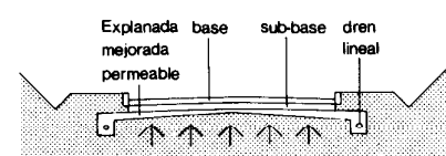
Drenaje de agua ascendente Sección transversal
