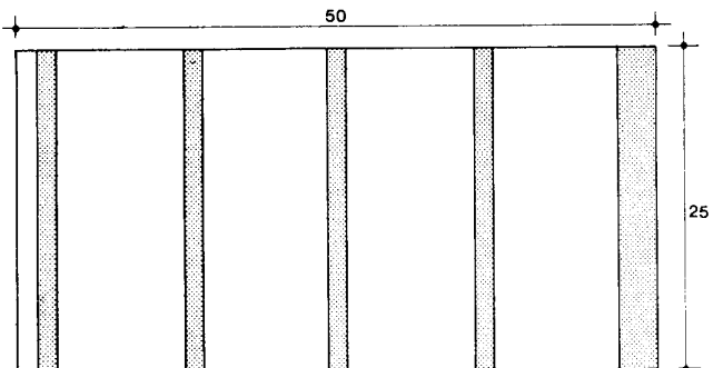
Sección vertical
