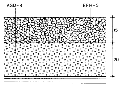
Sección transversal
