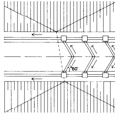
Planta Paso de desmote a terraplén
