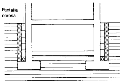
Sección vertical
