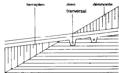
Sección longitudinal
