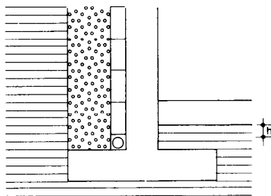
Sección vertical
