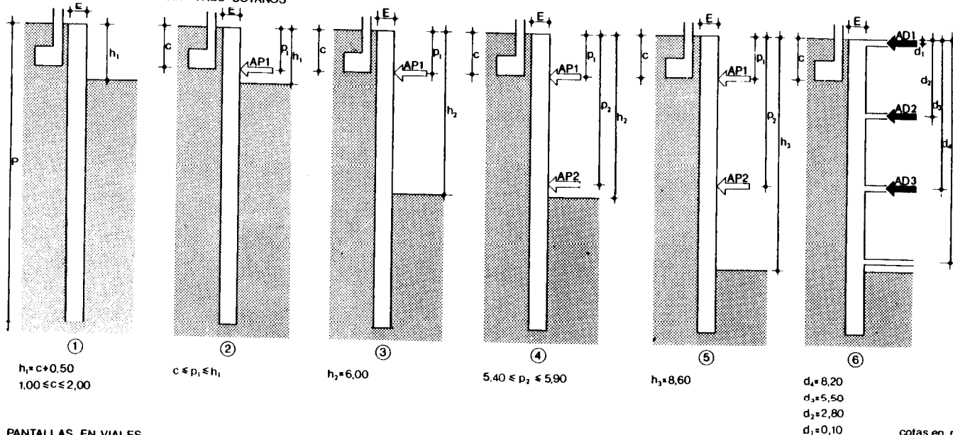
PANTALLAS EN VIALES FASES DE EJECUCION PARA TRES SOTANOS
