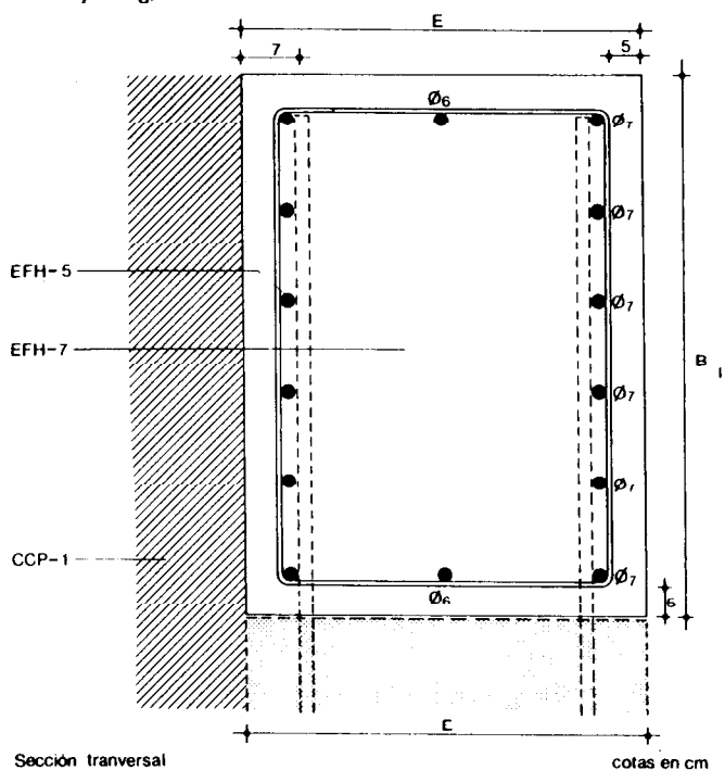
CCP-8 Viga de atado de paneles · E · B · T · n \varnothing_6 · EFH-5 Armadura de acero m \varnothing_7 · \varnothing_8 .
