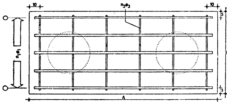
Sección
