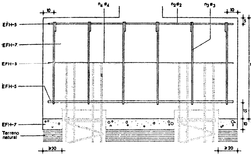
Sección
