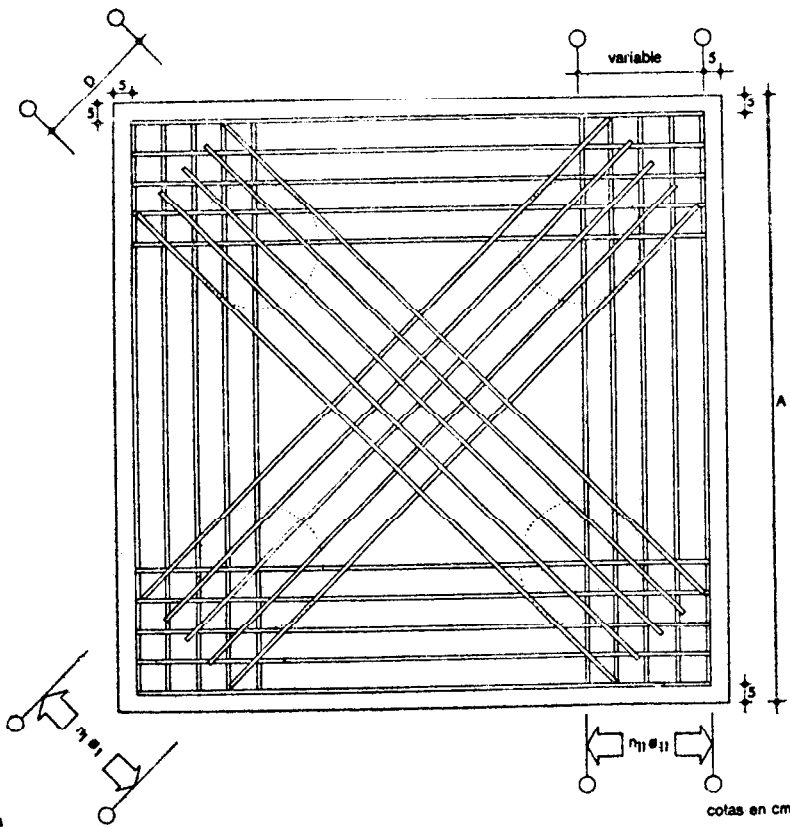
Planta
