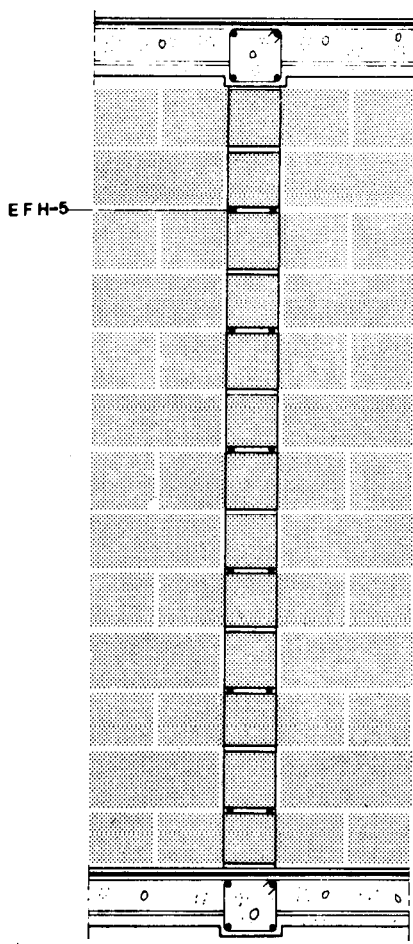
Sección B-B
