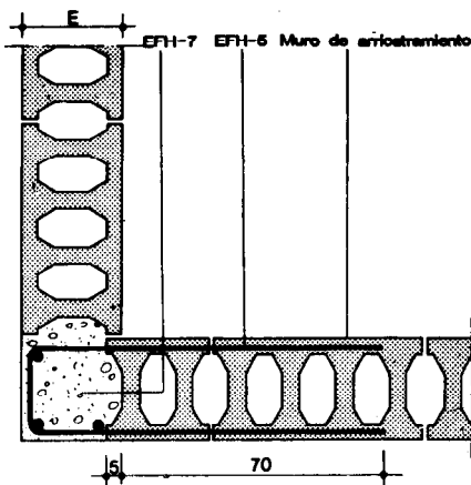
Hiladas pares
