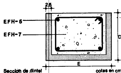
Sección de dintel
