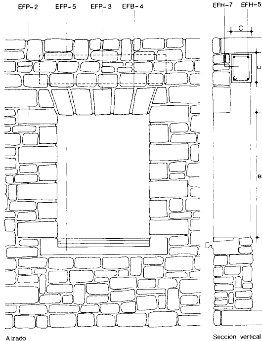
Alzado
