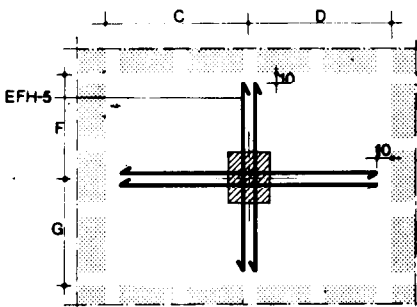
Planta cotas en cm
