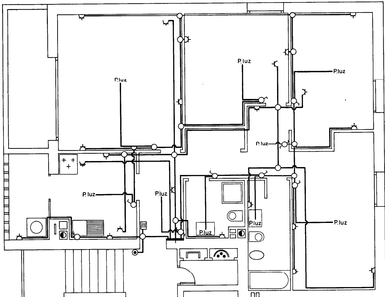
Planta de vivienda
