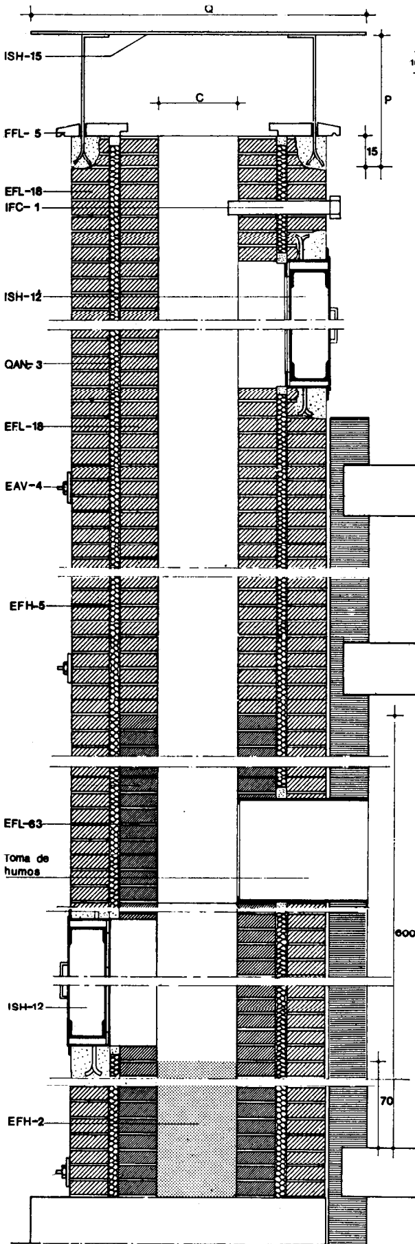
cotas en cm
