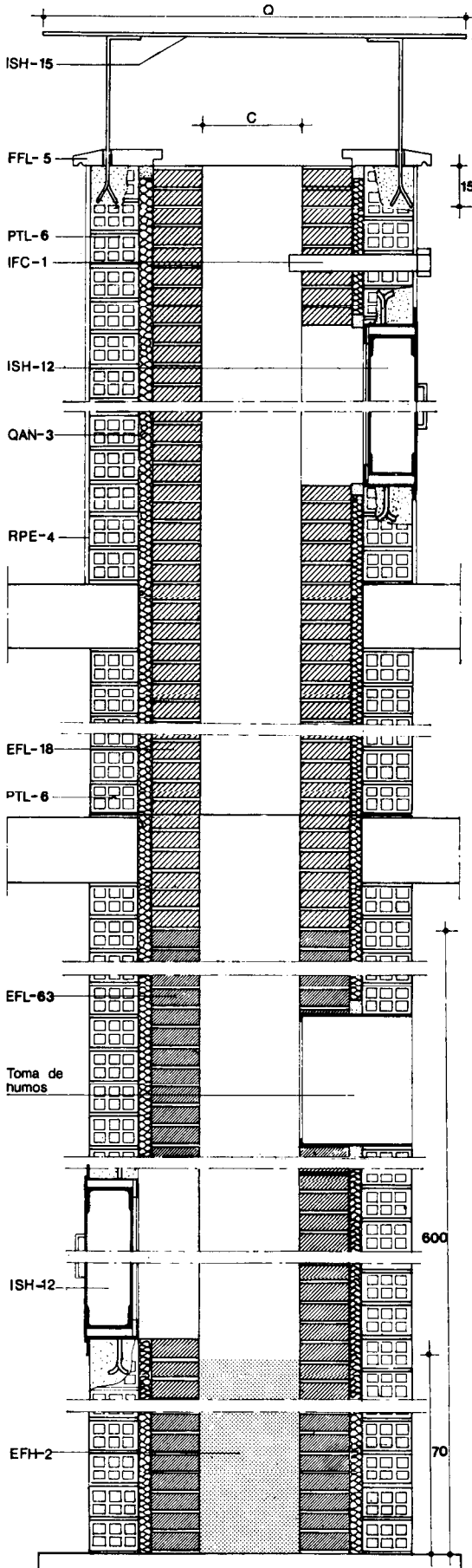
Paño de chimenea por forjado
