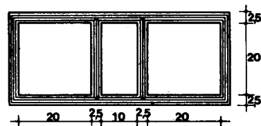
Planta
