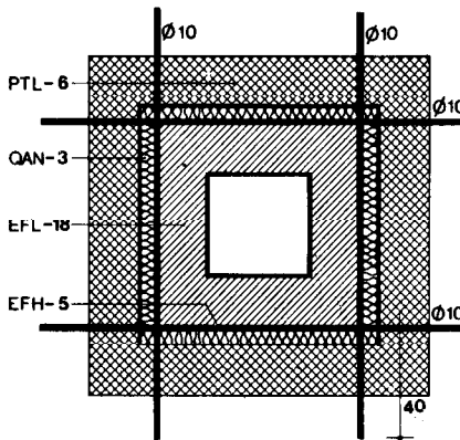
Paño de chimenea por forjado
