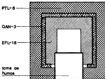
Sección por toma de humos
