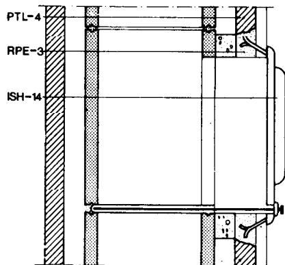
Sección
