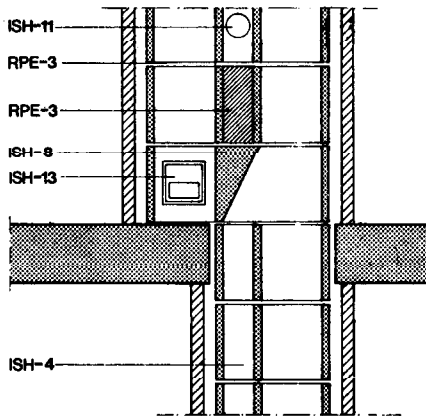
Detalle 1ª planta
