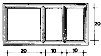
Planta
