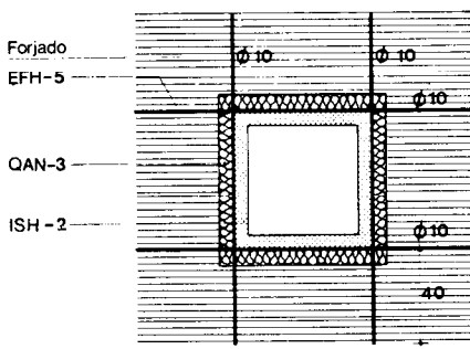
Paso de chimenea por forjado
