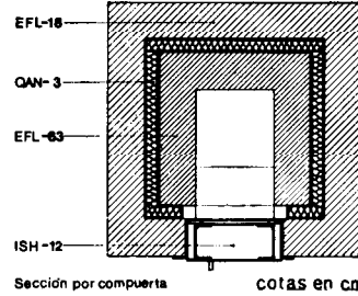
cotas en cm
