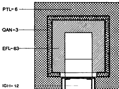
Sección por compuerta
