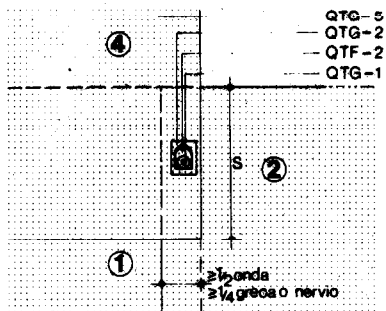
Detalle A-A
