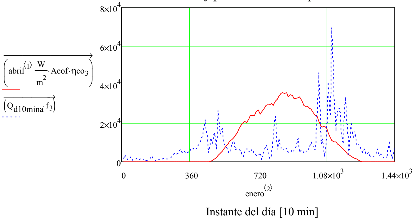
Figura 71: Radiación útil y potencia térmica aportada en Abril
