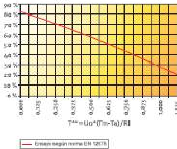
RENDIMIENTO CAPTADOR HR 2.02 4V
