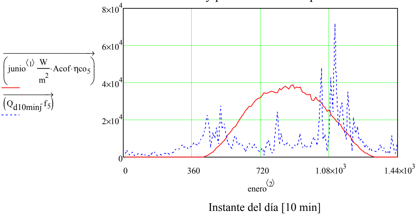
Figura 73: Radiación útil y potencia térmica aportada en Junio
