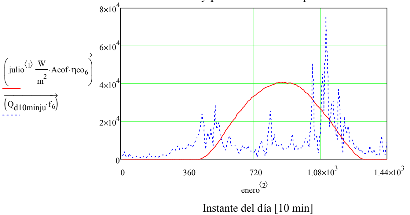
Figura 74: Radiación útil y potencia térmica aportada en Julio
