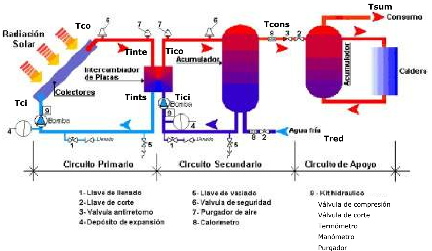
Figura 24: Componentes de una instalación solar
