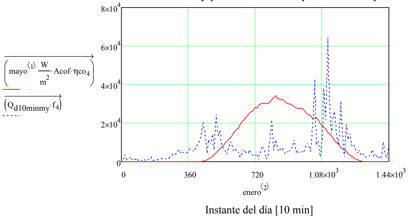
Figura 72: Radiación útil y potencia térmica aportada en Mayo
