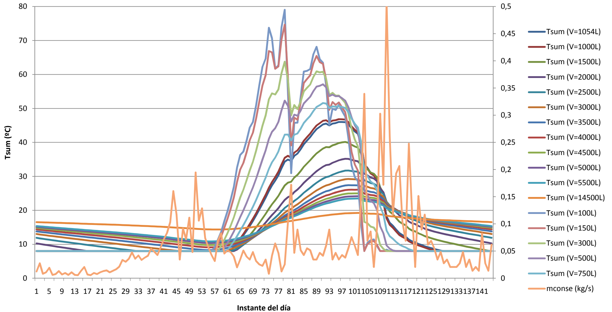
Figura 125: Evolución de la temperatura de suministro en Enero para diferentes volúmenes de tanque
