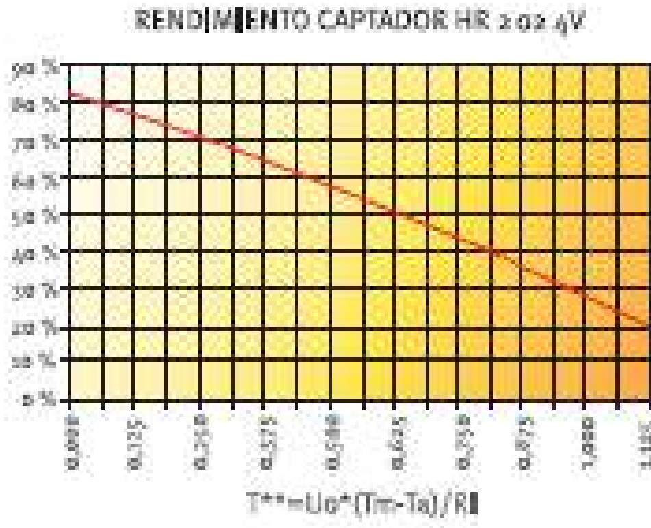
Figura 23: Recta de normalización del colector solar proyectado
