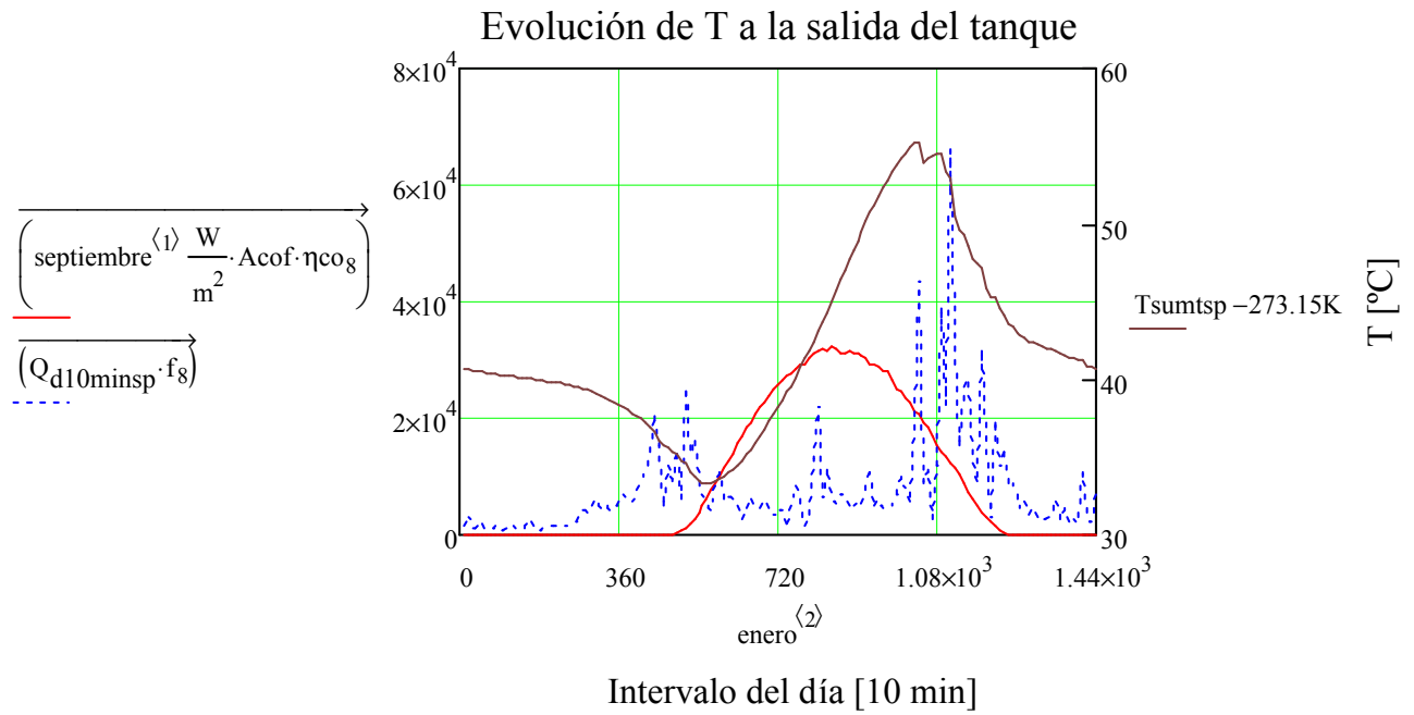
Figura 89: Evolución de la temperatura de consumo en Septiembre
