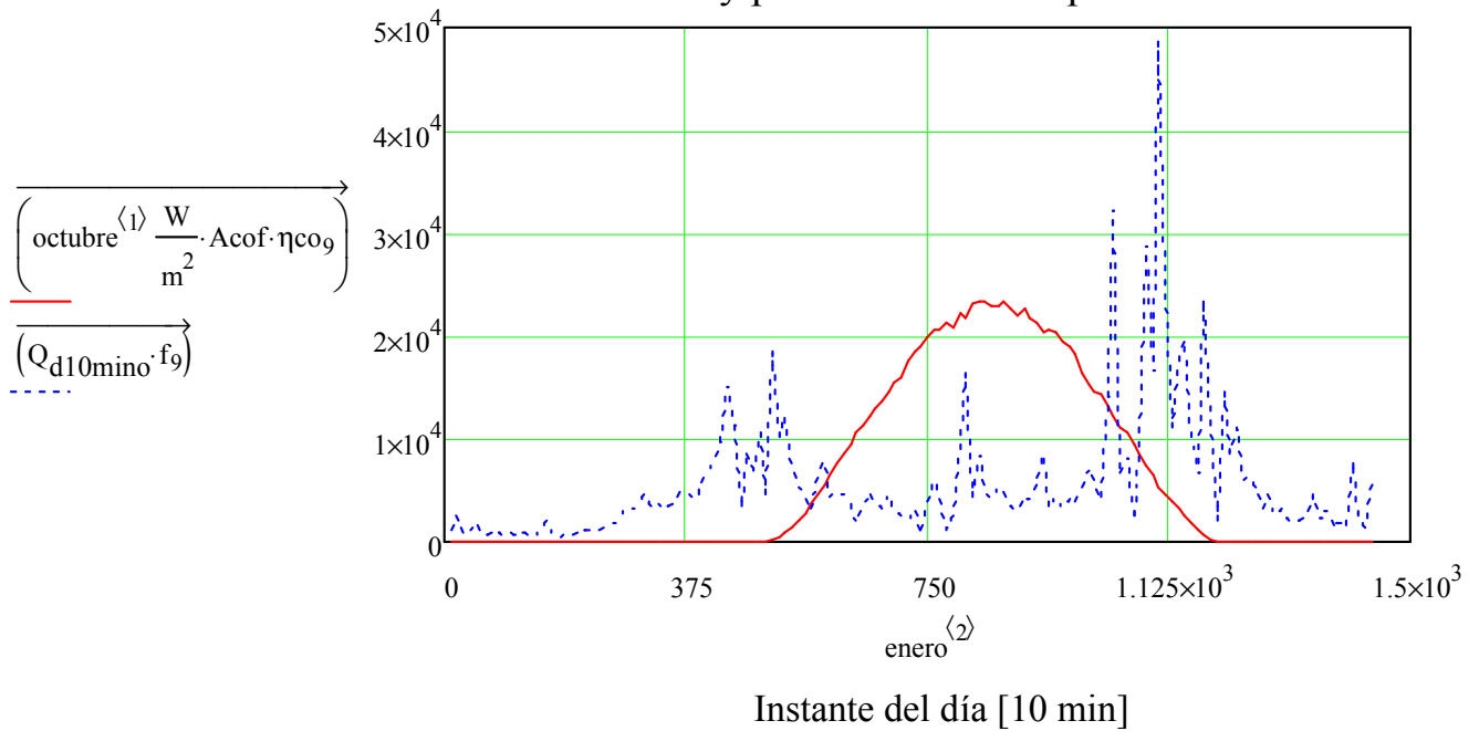
Figura 77: Radiación útil y potencia térmica aportada en Octubre
