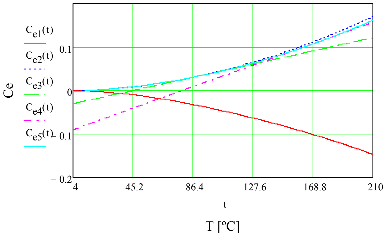
Figura 67: Coeficientes de expansión en función de la temperatura
