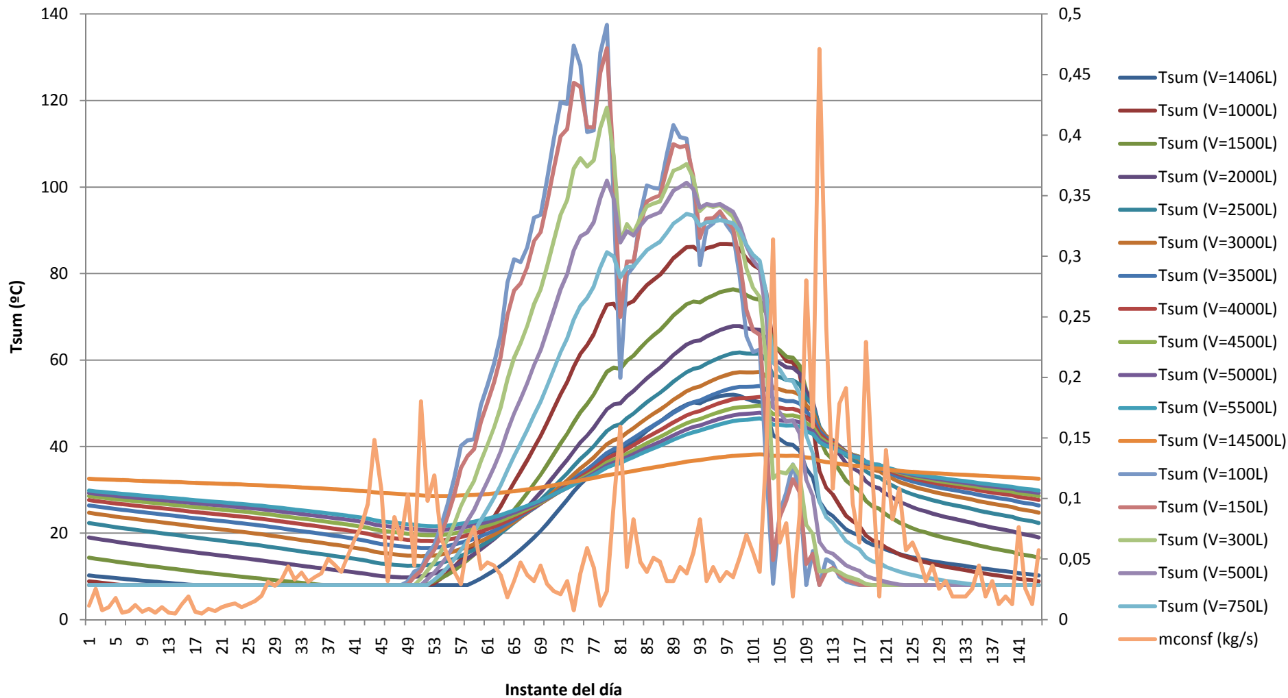
Figura 126: Evolución de la temperatura de suministro en Febrero para diferentes volúmenes de tanque
