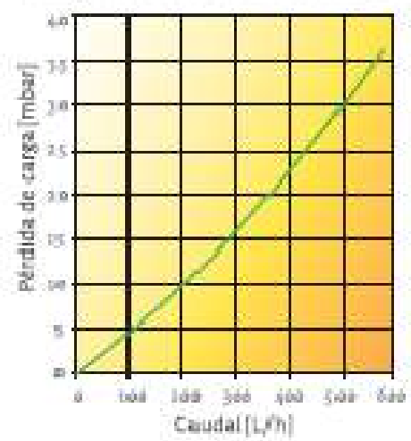
PÉRDIDA DE CARGA CAPTADOR HR 2.02 4V
