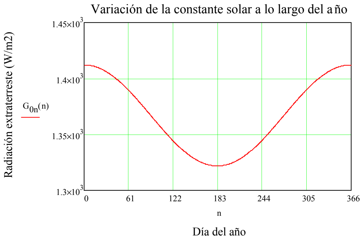
Figura 6: Variación de la constante solar a lo largo del año
