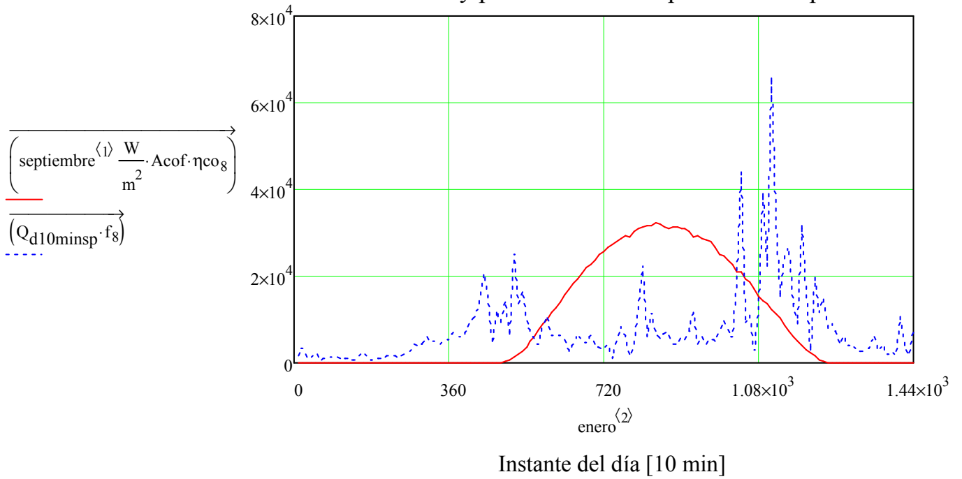
Figura 76: Radiación útil y potencia térmica aportada en Septiembre
