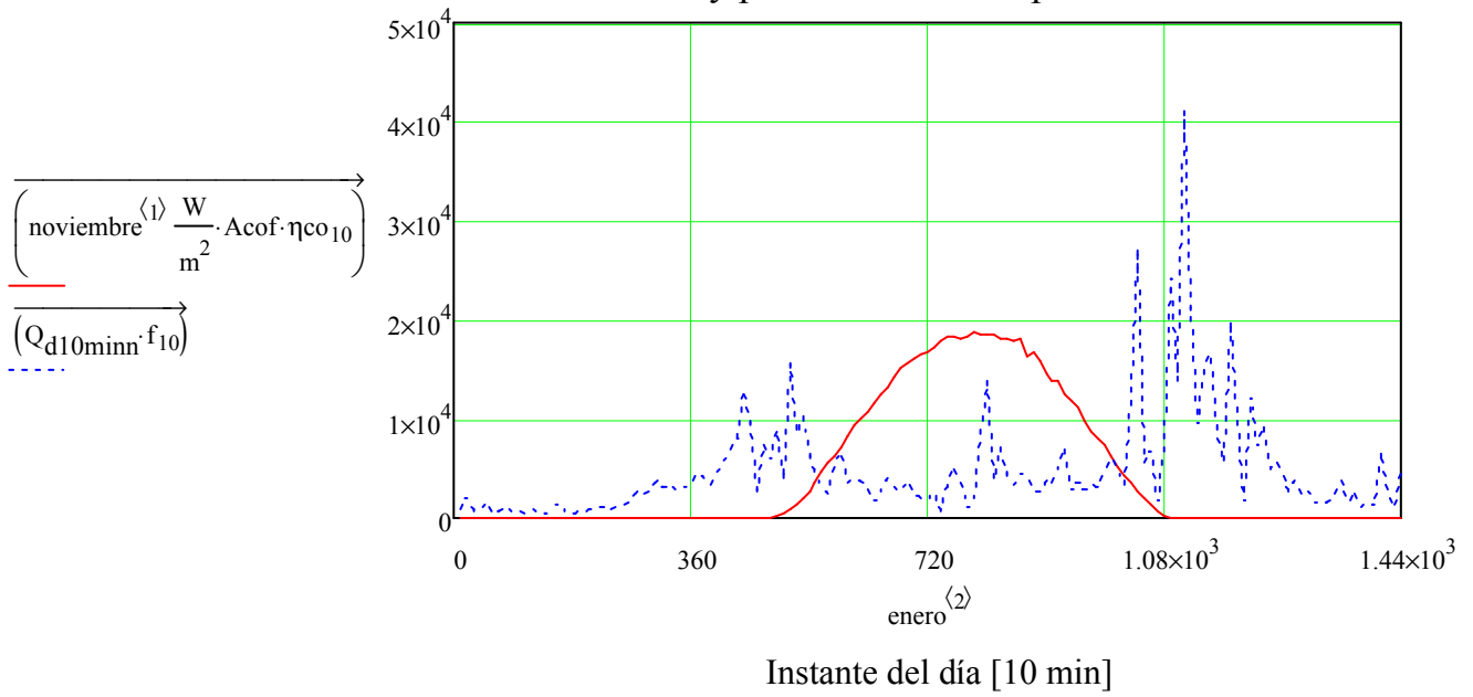
Figura 78: Radiación útil y potencia térmica aportada en Noviembre
