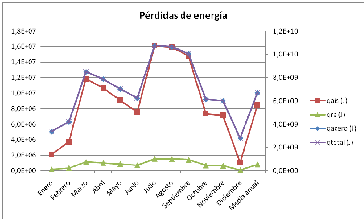
Figura 51: Variación mensual de las pérdidas de energía
