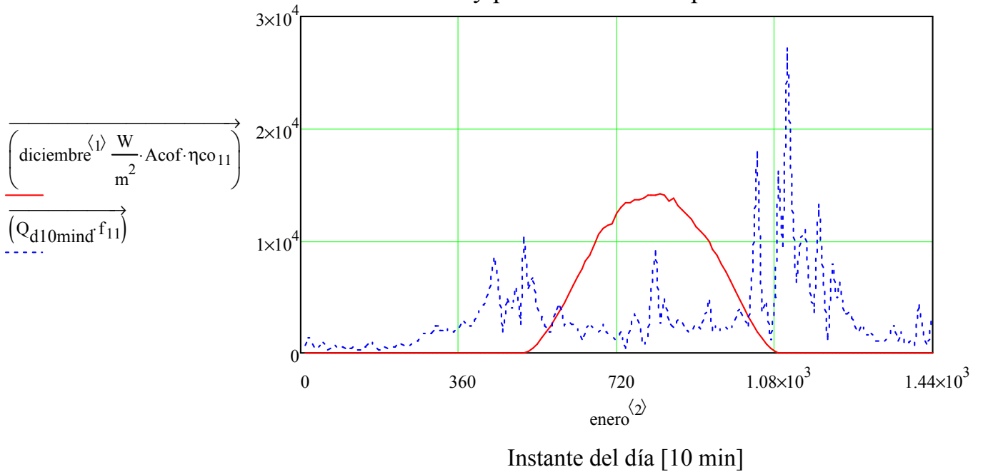
Figura 79: Radiación útil y potencia térmica aportada en Diciembre
