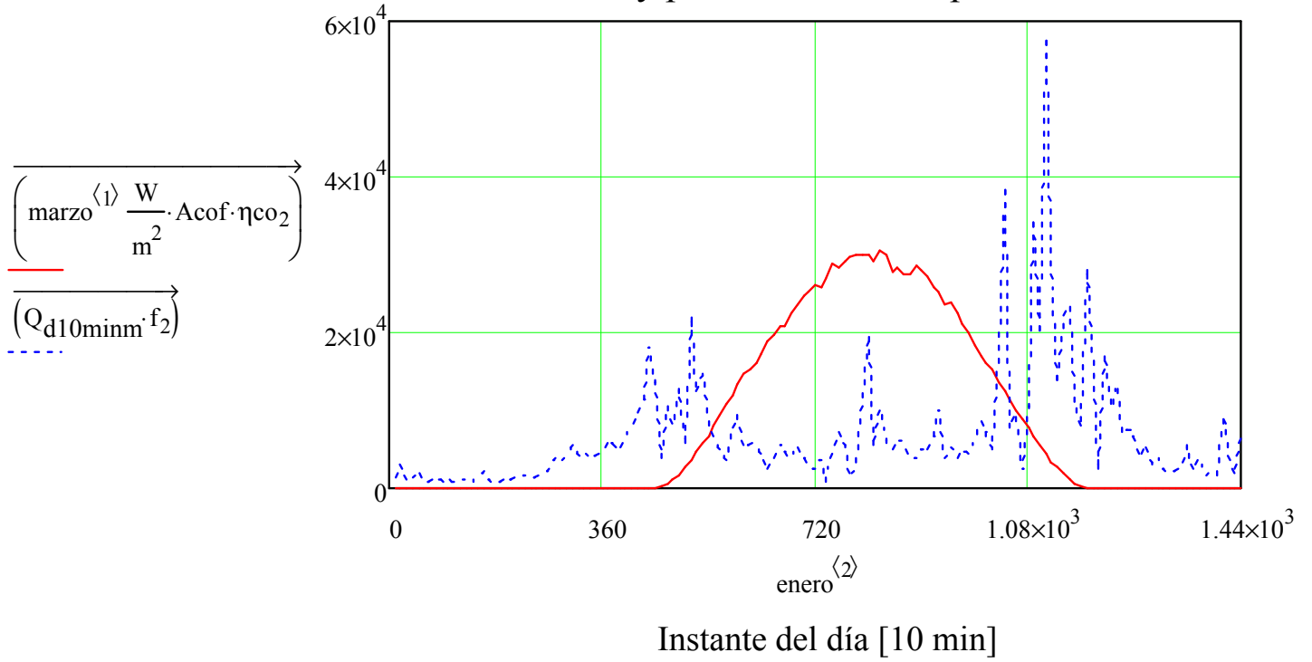
Figura 70: Radiación útil y potencia térmica aportada en Marzo
