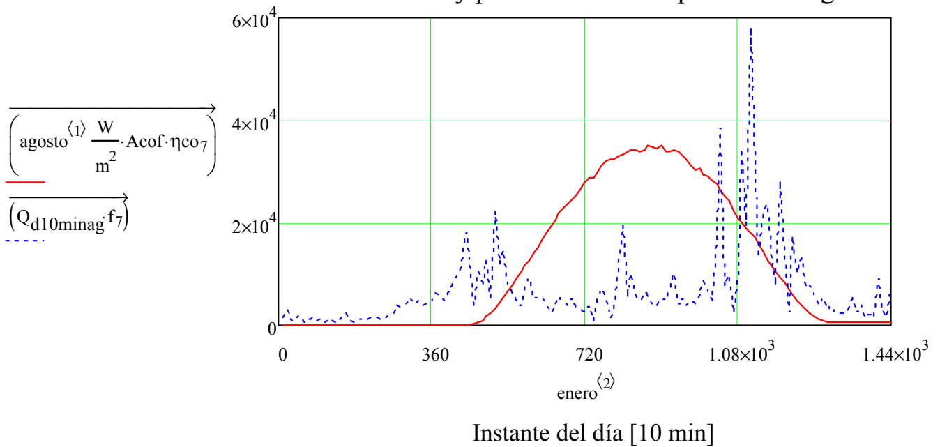
Figura 75: Radiación útil y potencia térmica aportada en Agosto
