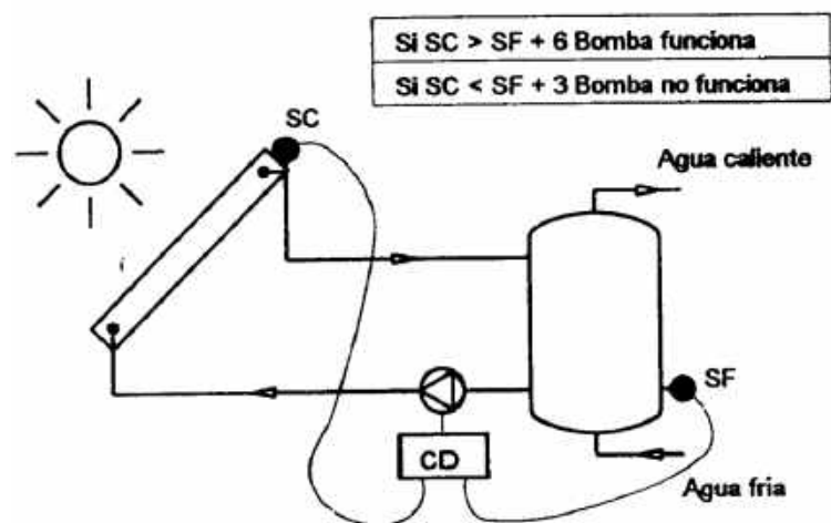
Figura 6: Esquema instalación por circulación forzada.
