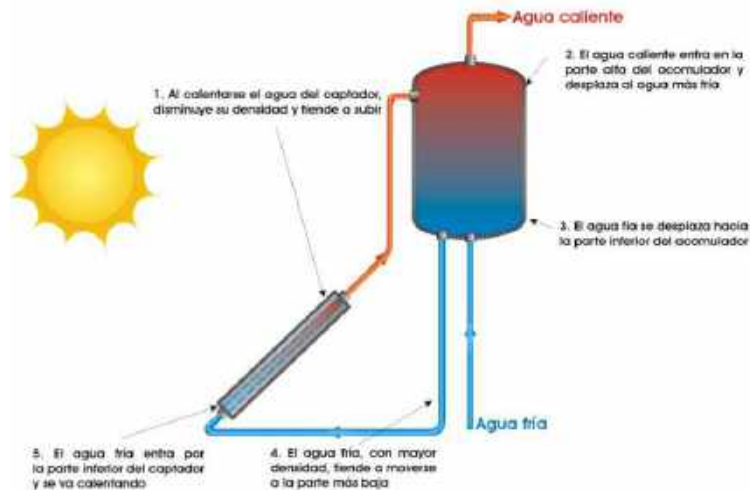
Figura 5: Instalación con acumulador.
