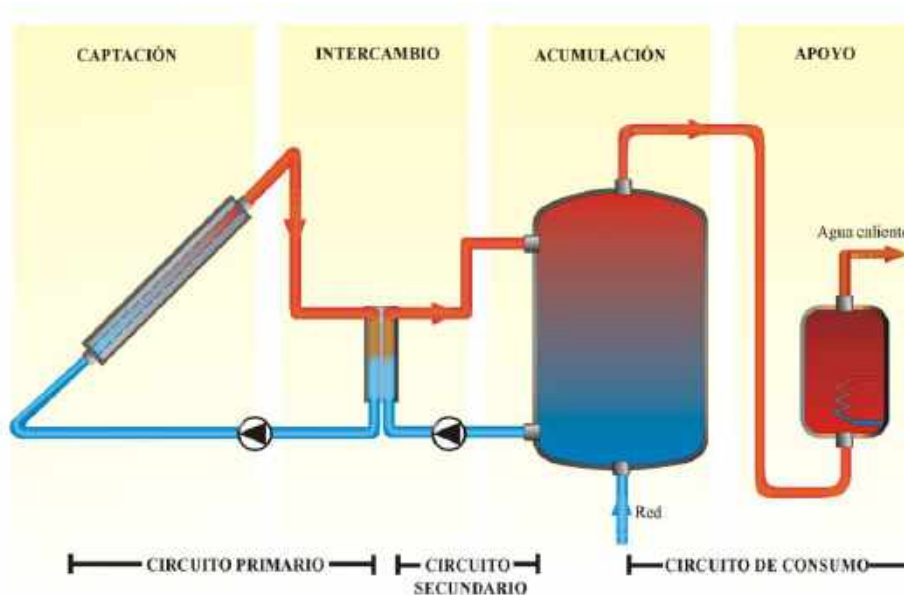
Figura 4: Esquema de la instalación.
