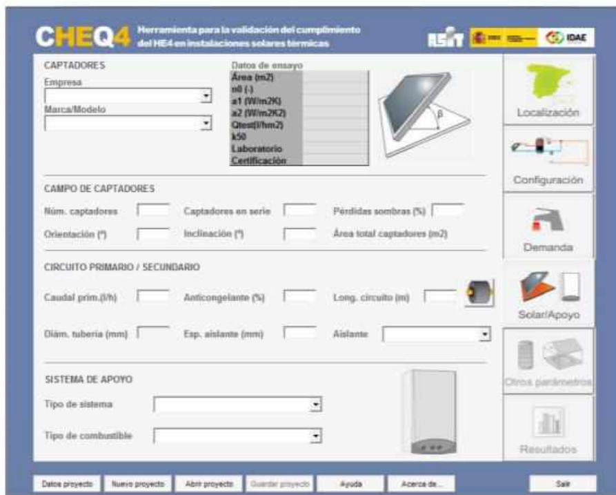
Figura 13: Parámetros del sistema. Solar/Apoyo.
