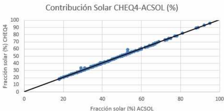
Gráfica 1: Contribución solar CHEQ4-ACSOL (%).
