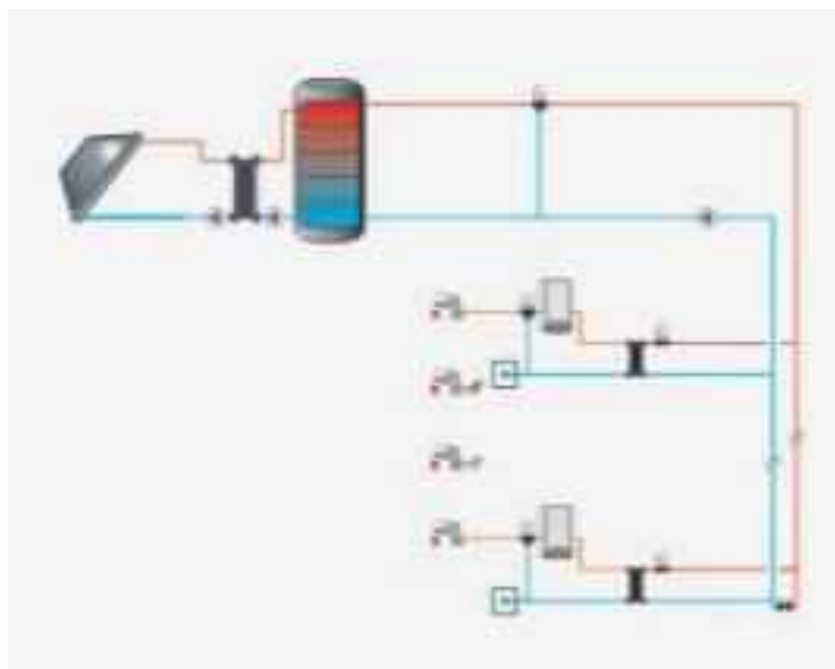
Figura 10: Instalación para consumo múltiple con intercambio distribuido.
