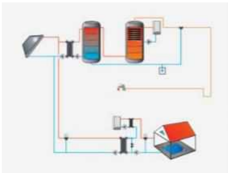
Figura 16: Instalación para consumo único con intercambiador y piscina cubierta.
