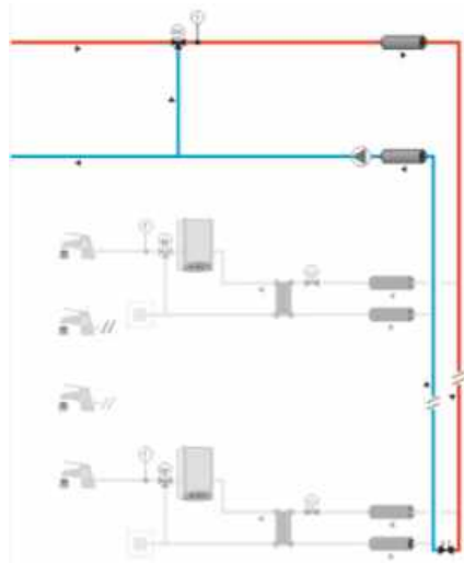
Figura 17: Circuito y distribución.
