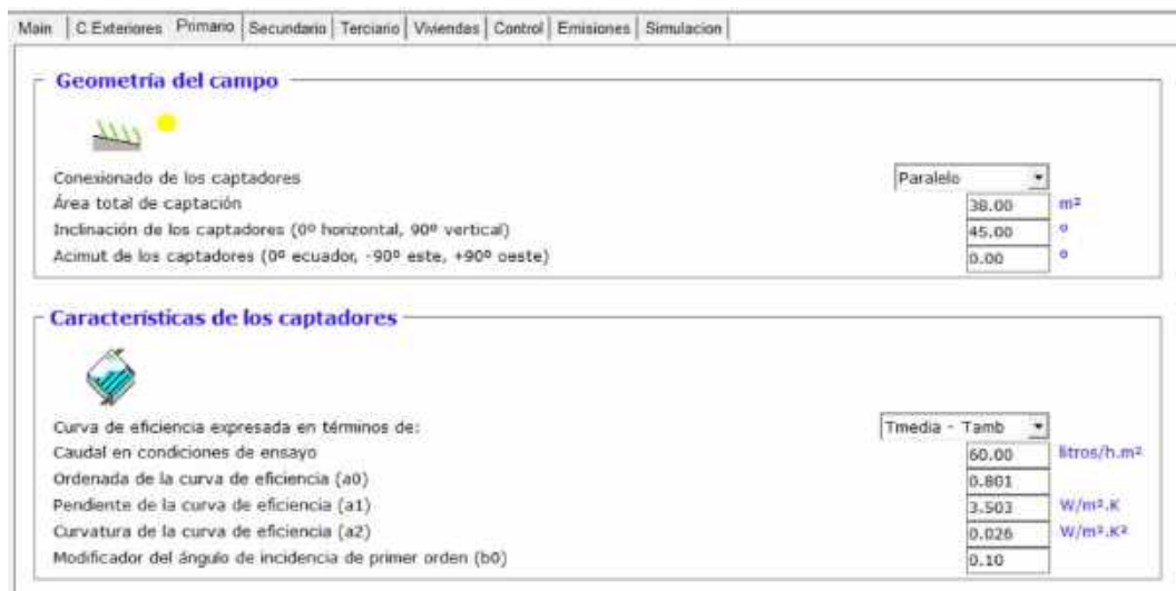
Figura 27: Pantalla circuito primario (1).
